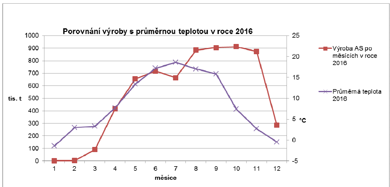
Graf č. 3: Porovnání výroby asfaltových směsí s průměrnou teplotou v roce 2016
